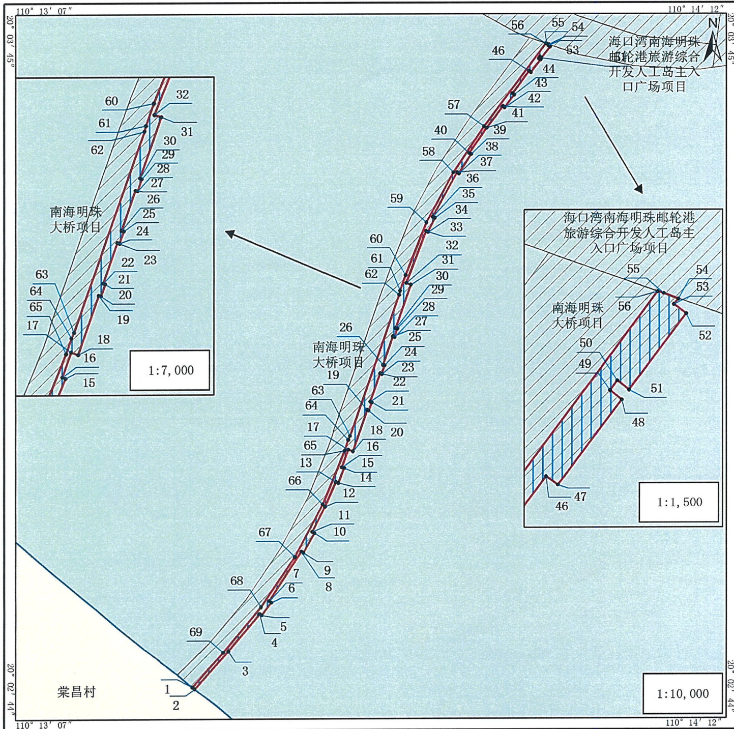
南海明珠大桥（临时栈桥）项目续期用海宗海界址图
